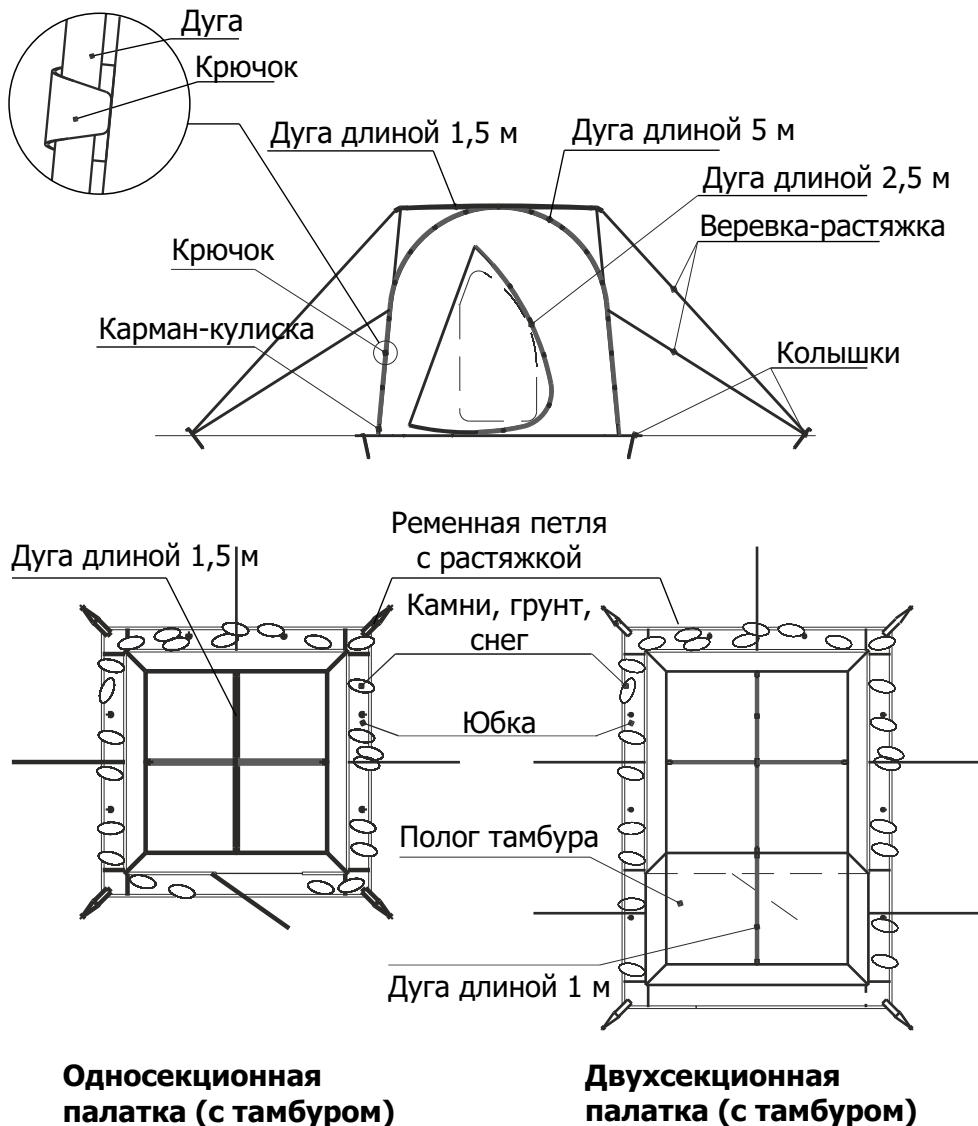
Рис. 3 Схема монтажа бани-палатки
